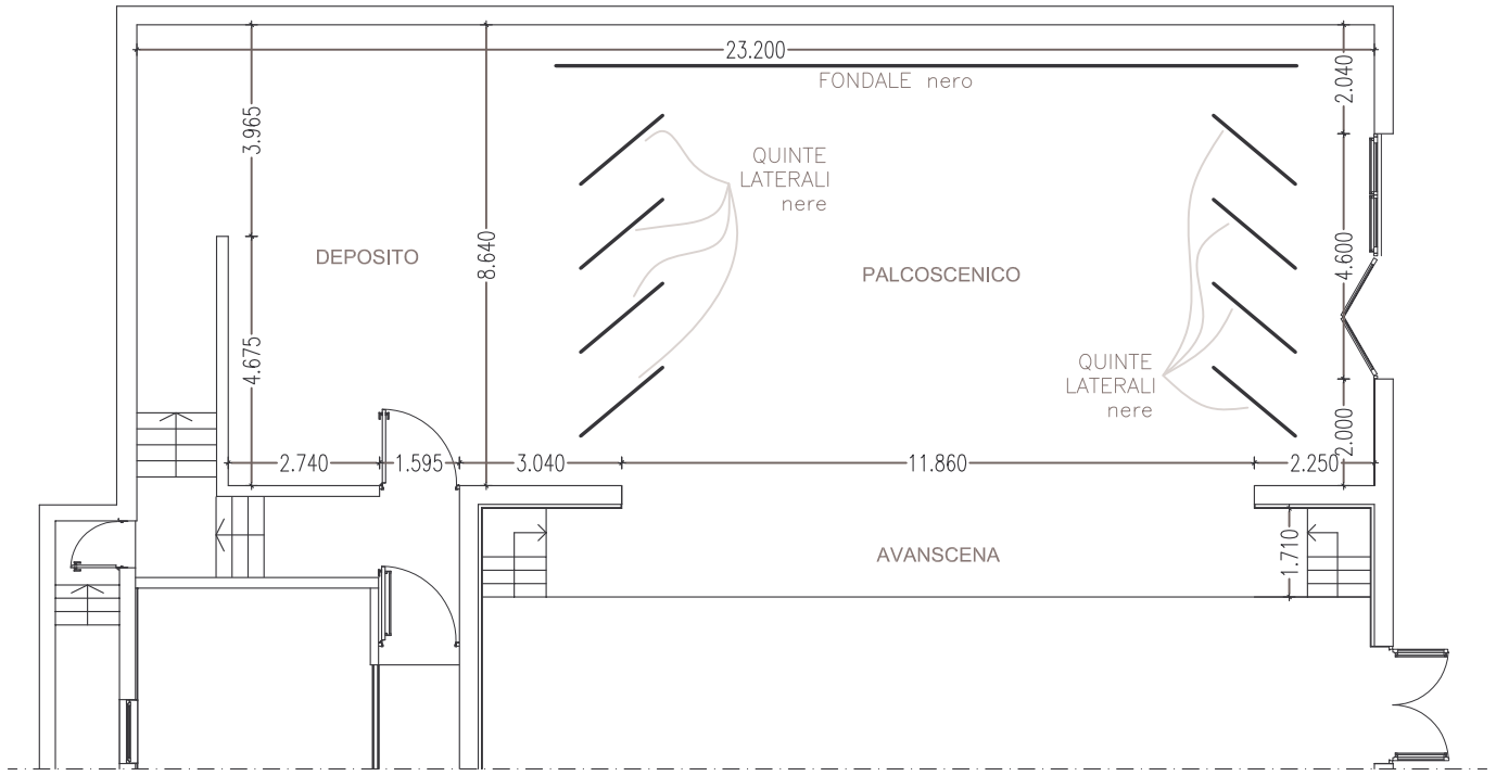
PIANTA PAVIMENTO PALCOSCENICO
