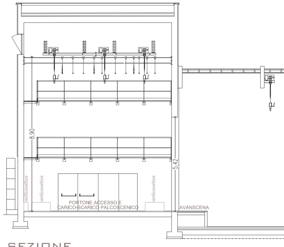
SEZIONE
